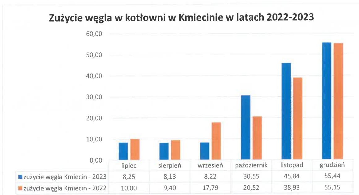
Wykres 22 Zużycie węgla na kotłowni w Kmiecinie przy ulicy Łąkowej w latach 2022 - 2023
