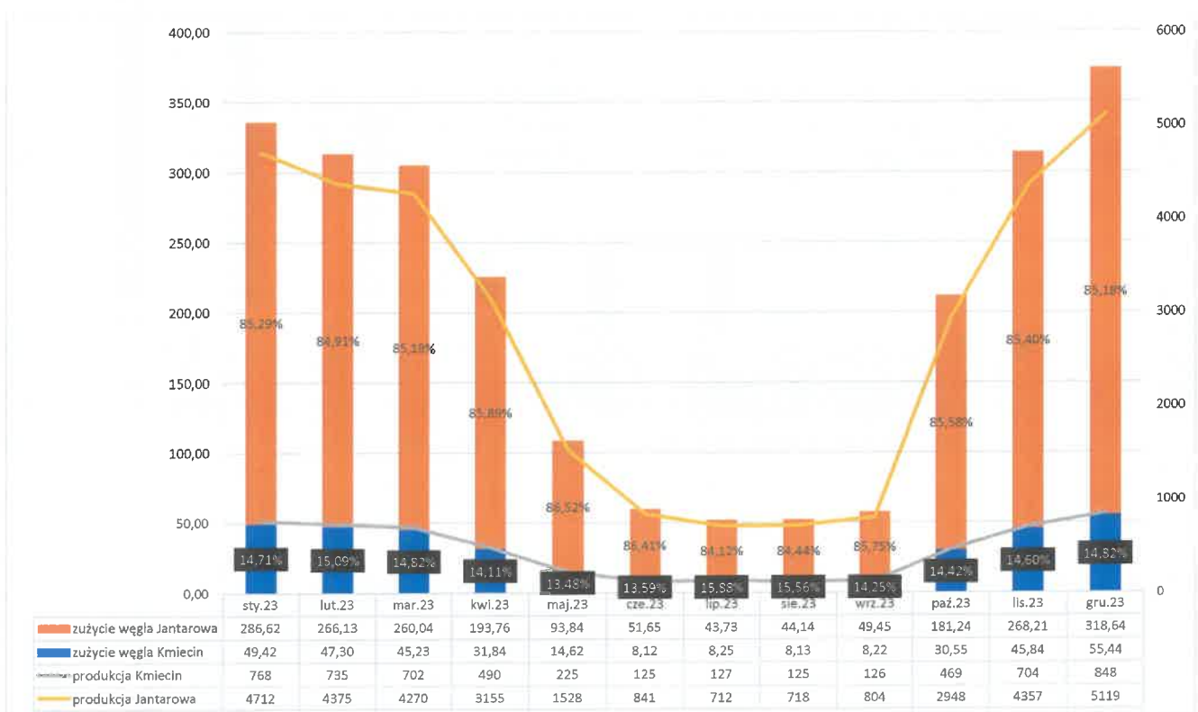
Wykres 21 Zużycie węgla na kotłowniach oraz ilość wyprodukowanych GJ w 2023 r.
