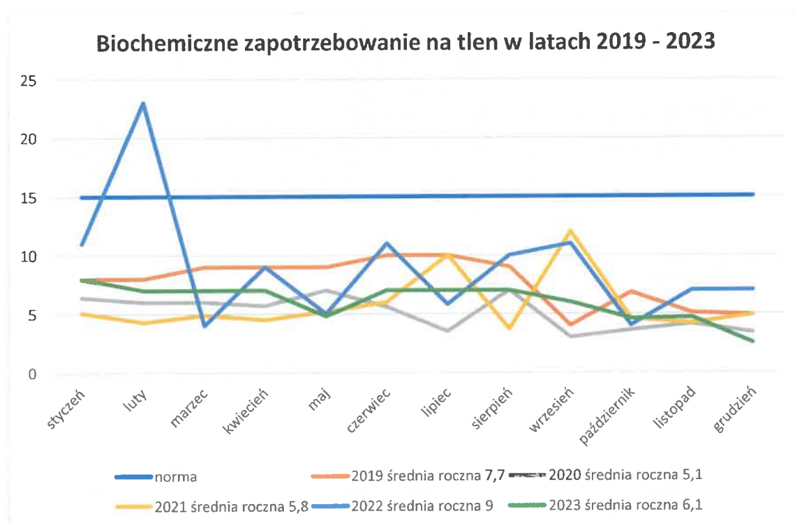
Wykres 1 Biochemiczne zużycie tlenu w latach 2019 – 2023 – BZT5
