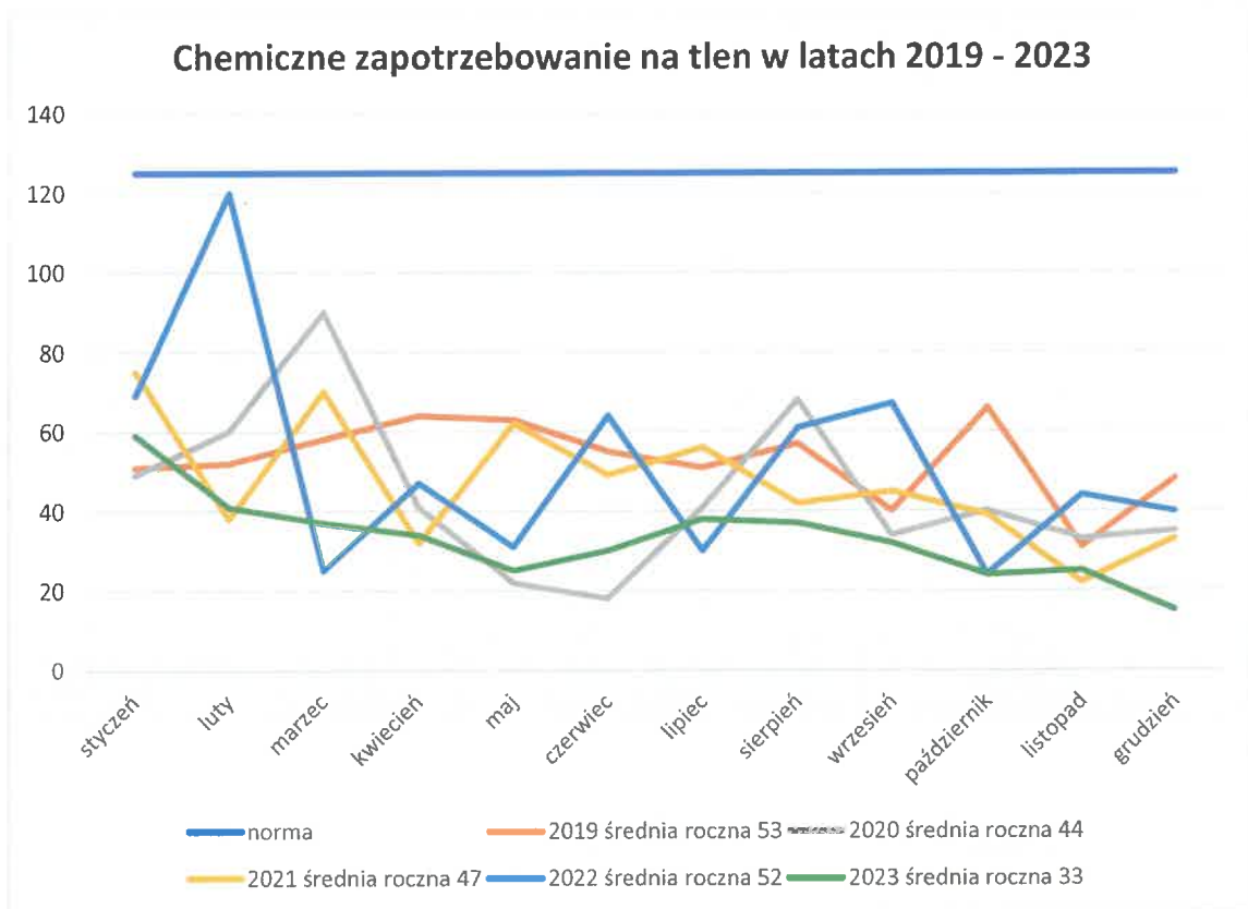
Wykres 2 Chemiczne zapotrzebowanie tlenu w latach 2019 -2023 ChZT
