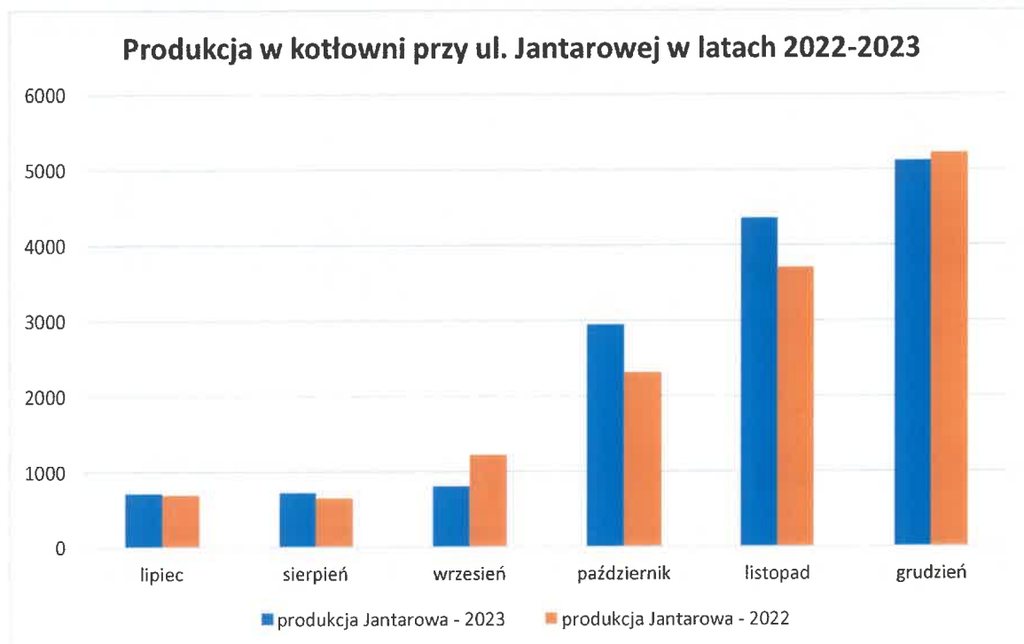
Wykres 25 Ilość wyprodukowanych GJ w kotłowni w Nowym Dworze Gdańskim przy ulicy Jantarowej w latach 2022 - 2023
