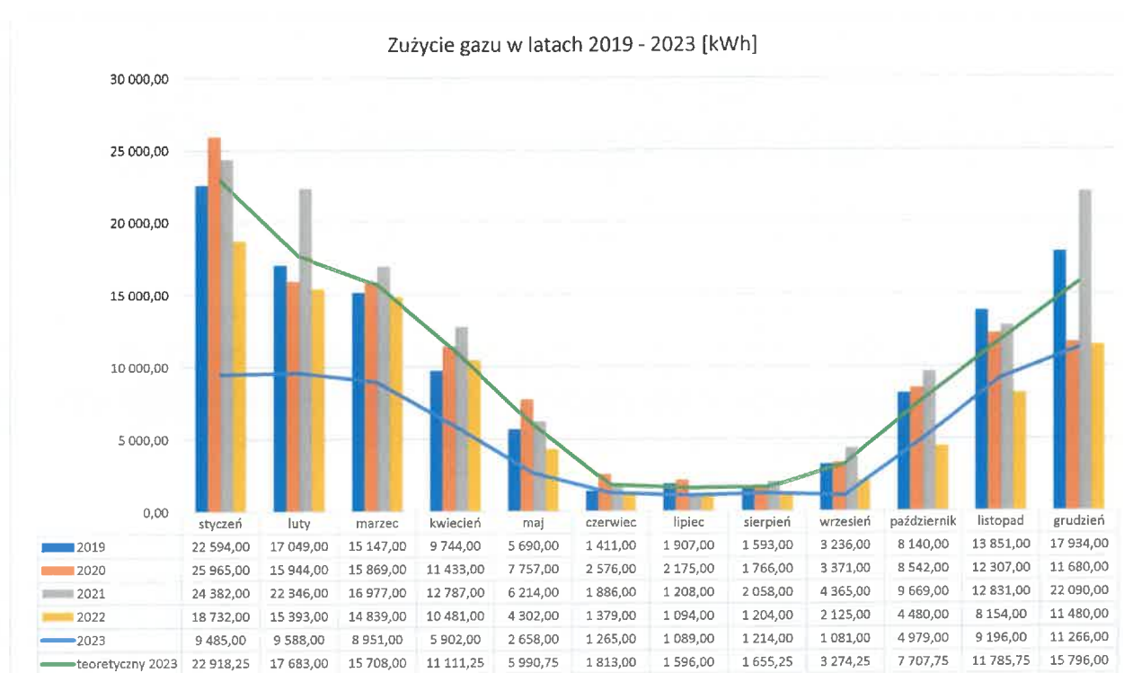
Wykres 16 Zużycie gazu w latach 2019 - 2023 w kWh
