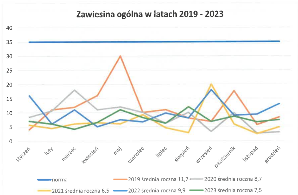
Wykres 3 Zawiesina ogólna w latach 2019 - 2023
