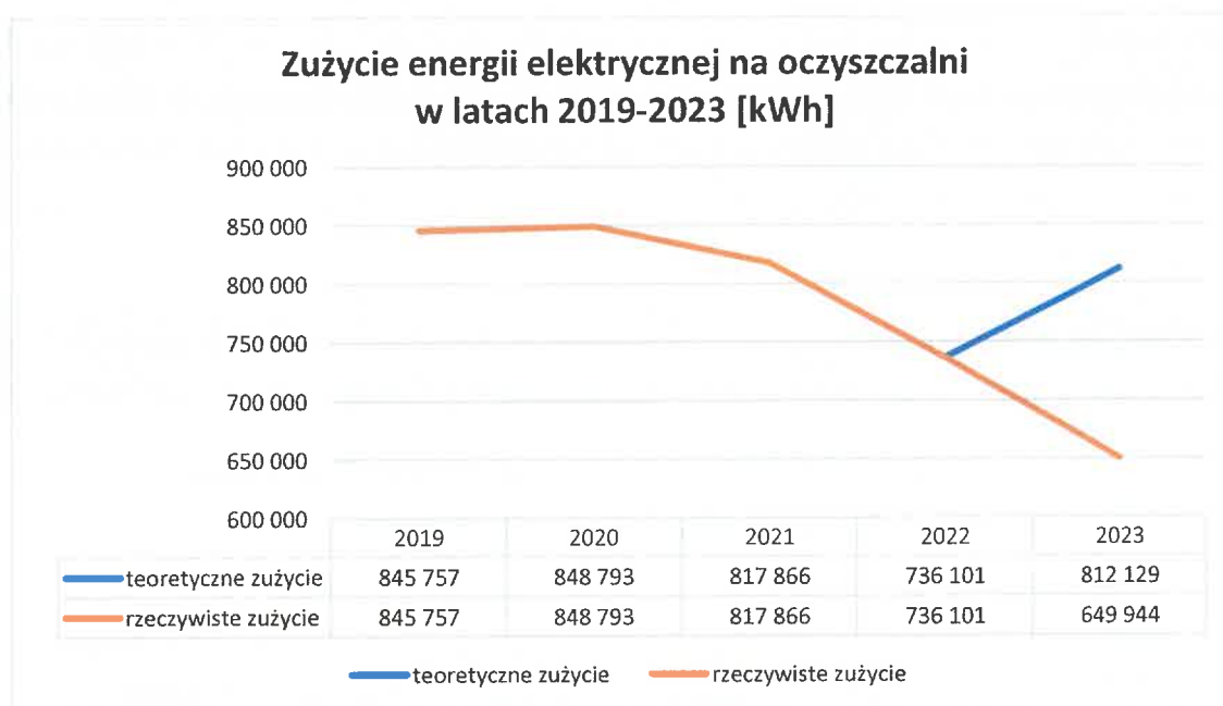
Wykres 14 Zużycie energii elektrycznej na oczyszczalni ścieków w latach 2019 -2023 [kWh]
