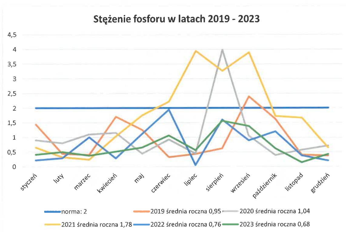
Wykres 5 Stężenie fosforu w latach 2019 - 2023
